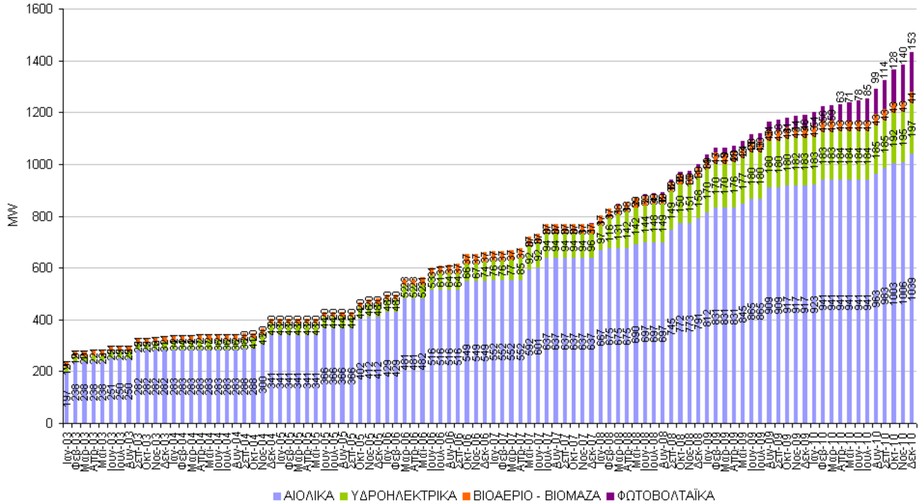
2003 – 2010 ΕΓΚΑΤΕΣΤΗΜΕΝΗ ΙΣΧΥΣ (ΜW) ΜΟΝΑΔΩΝ ΑΠΕ ΣΕ ΛΕΙΤΟΥΡΓΙΑ ΣΤΟ ΔΙΑΣΥΝΔΕΔΕΜΕΝΟ ΣΥΣΤΗΜΑ (Άρθρο 9 Ν.3468/2006)
