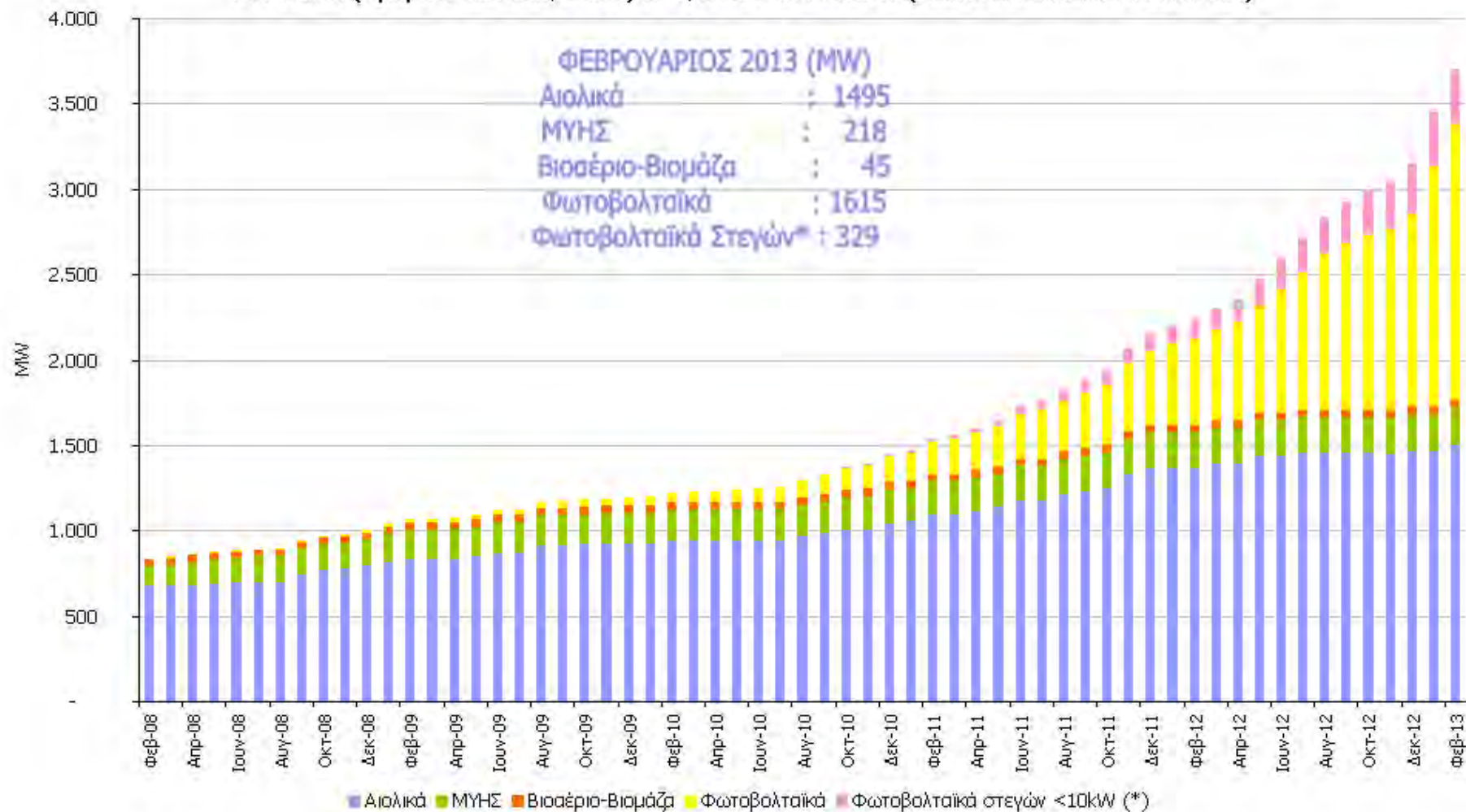
2008 – 2013 ΕΓΚΑΤΕΣΤΗΜΕΝΗ ΙΣΧΥΣ (MW) ΜΟΝΑΔΩΝ ΑΠΕ ΣΕ ΛΕΙΤΟΥΡΓΙΑ ΣΤΟ ΔΙΑΣΥΝΔΕΔΕΜΕΝΟ ΣΥΣΤΗΜΑ (Άρθρο 9 Ν.3468/2006) & Φ/Β ΣΤΕΓΩΝ < 10kW (*ΔΙΑΣΥΝΔΕΔΕΜΕΝΟ ΚΑΙ ΜΗ)
